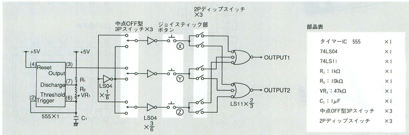
図2 回路図
